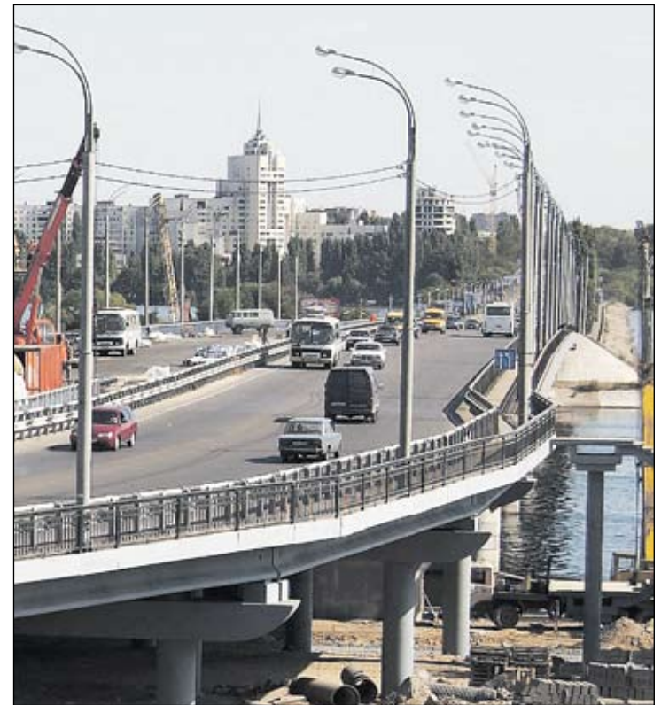
Все колебания пролетов конструкции фиксировались специальными датчиками, закрепленными под мостом
