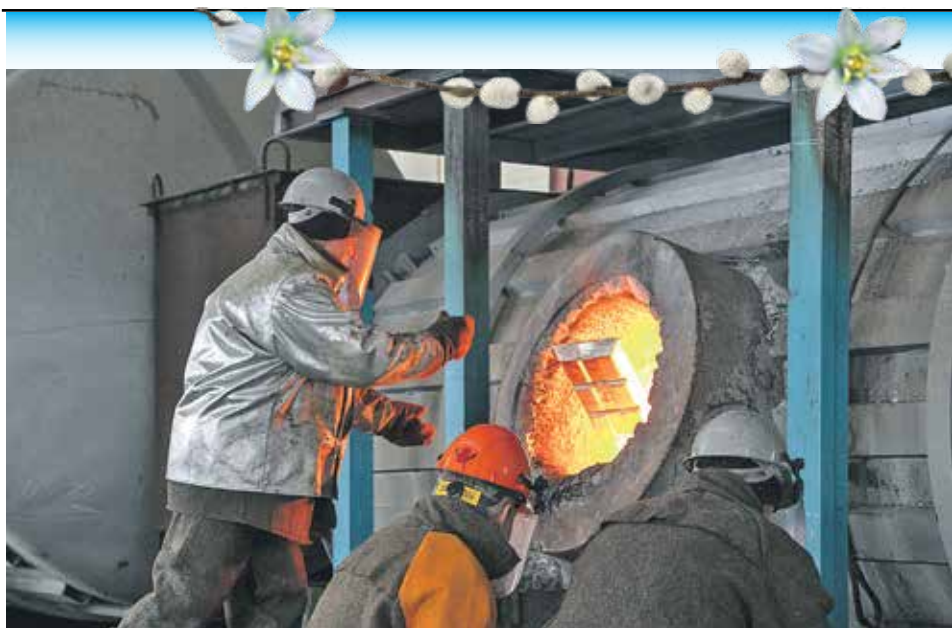
Колокола изготавливаются из специальной бронзы – подготовленного сплава меди (80 %) и олова (20 %). Температура плавления превышает 1100 °С
